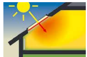
Η ακτινοβολία που εισέρχεται μέσω του υαλοπίνακα απορροφάται από το εσωτερικό κουρτινάκι. Αλλάζει μακροπρόθεσμα σε υπέρυθη ακτινοβολία (θερμότητα) η οποία δεν μπορεί να βγει έξω από τον υαλοπίνακα. Το κουρτινάκι εκπέμπει τη θερμότητα στο χώρο και λειτουργεί έτσι σαν θερμαντικό σώμα. Οδηγεί σε ανεπιθύμητη υπερθέρμανση των δωματίων, ιδιαίτερα αυτών που έχουν νότιο προσανατολισμό
